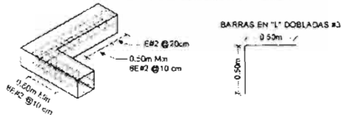
UNIÓN DE VIGA DE AMARRE EN ESQUINA
