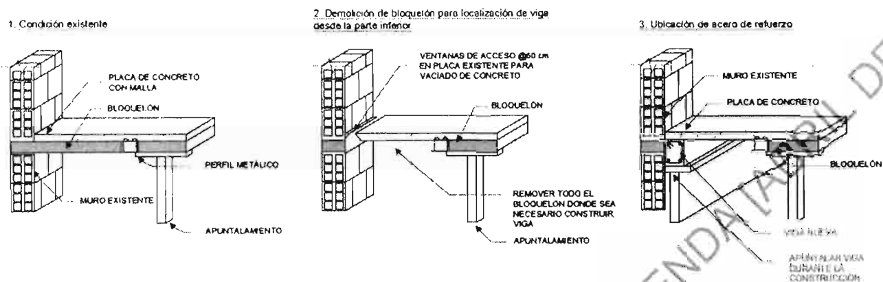
Figura A.3 -22 Construcción de nueva viga para dar rigidez al diafragma. Viga paralela a los perfiles metálicos.
