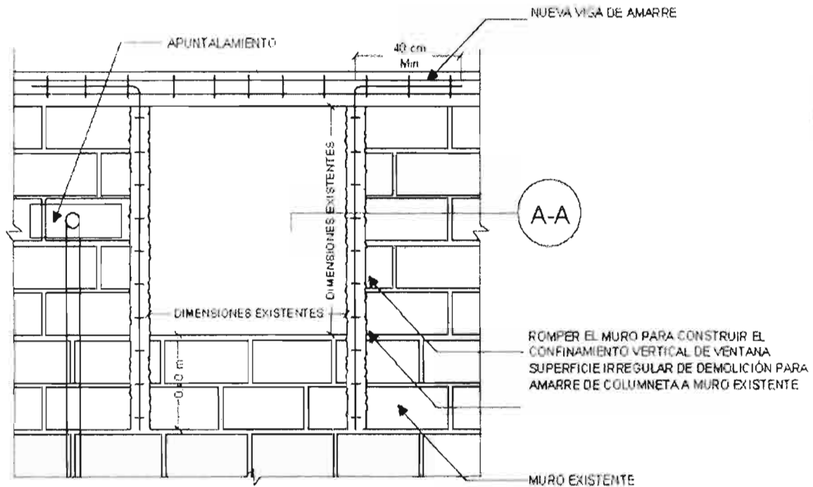
Figura A.3 -14 Refuerzo de vanos existentes.
