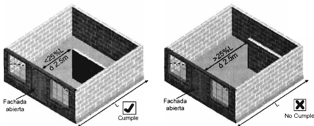
Figura 7.4-2 Chequeo parámetros para torsión
