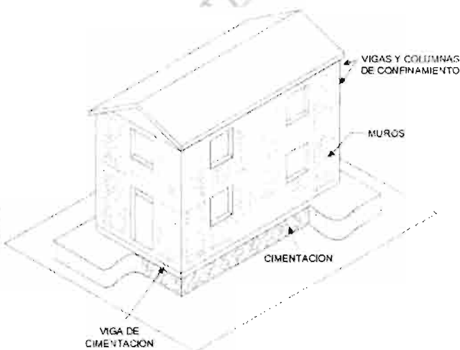
Figura 7.2-1 Elementos estructurales de una vivienda confinada
