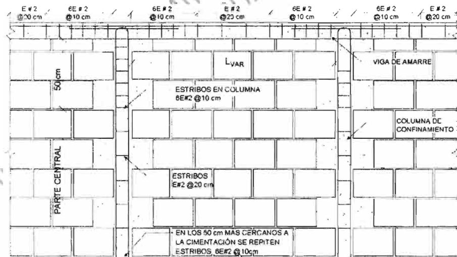
CONEXIÓN VIGA DE AMARRE EN ENCUENTRO DE TRES MUROS
