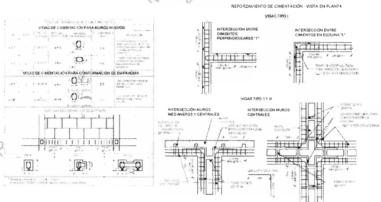
Figura A.3 -6 Despiece de nuevas vigas de cimentación para refuerzo de sistemas existentes.
