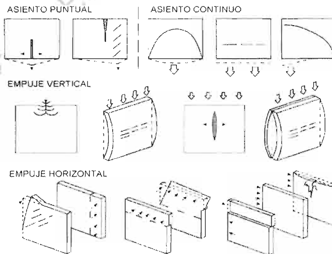
Figura 6-3 Tipos de fisuras
