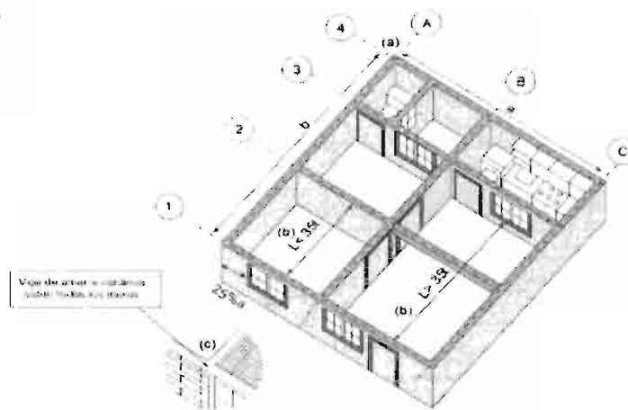
Figura 6.4.3-1 Chequeo por trayectoria de cargas.
