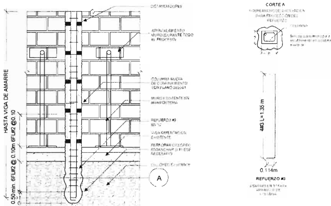
Figura A.3 -12 Anclaje de nueva columna de confinamiento a cimentación existente.
