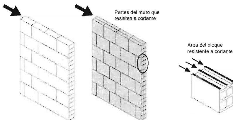
Figura 5-2 Área del bloque resistente a cortante
