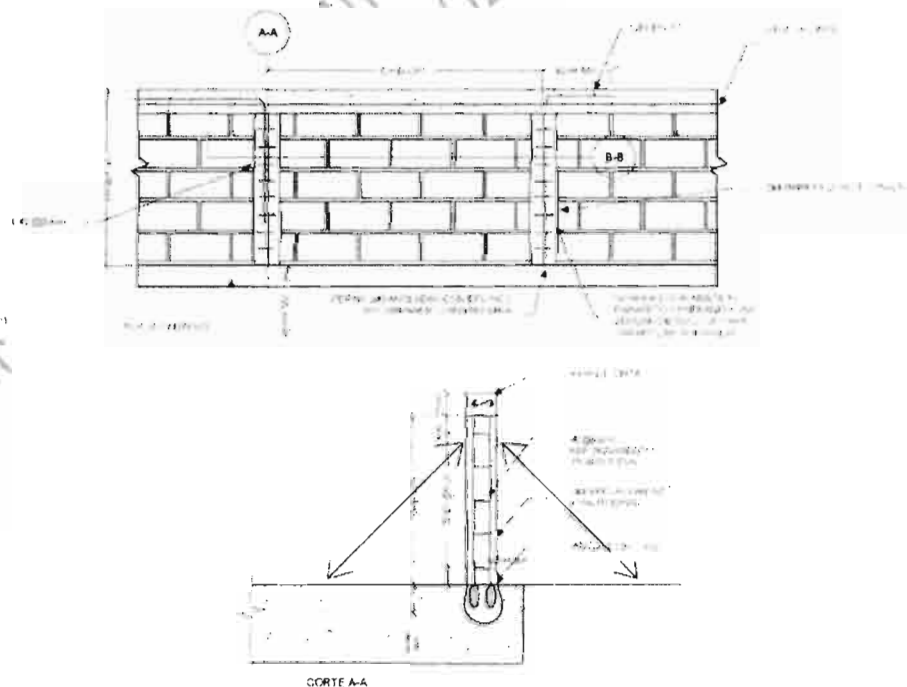
Figura A.3 -13 Refuerzo de parapeto existente.
