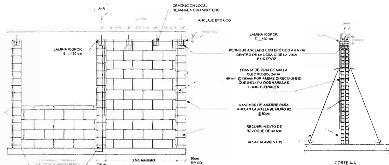
Figura A.3 -15 Dilatación de muros existentes.
