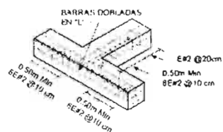
CONEXIÓN VIGA DE AMARRE EN ENCUENTRO DE TRES MUROS
