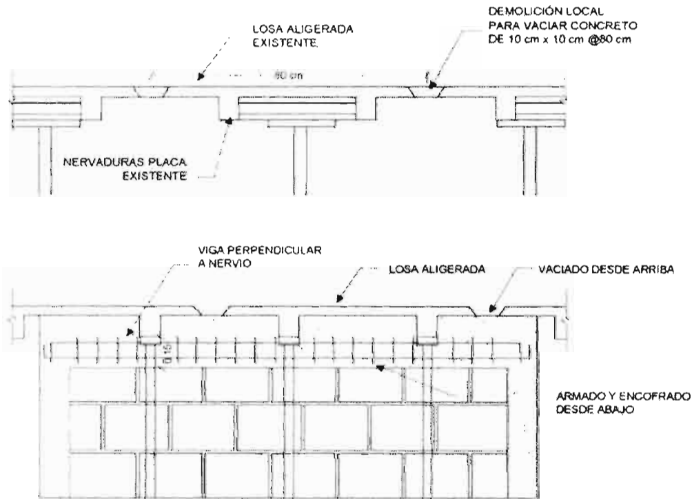
Figura A.3 -18 Conexión de muro nuevo a losa existente con nervios. Muro perpendicular a los nervios.
