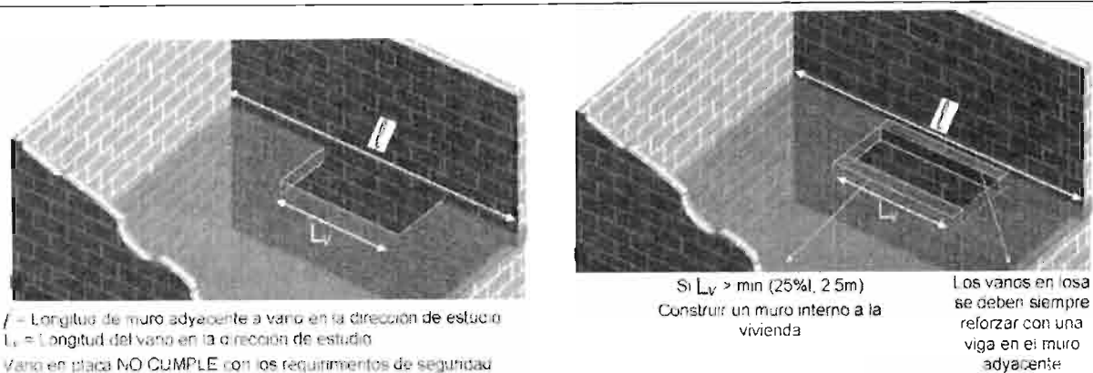
Figura 6.4-8 Vanos en placa
